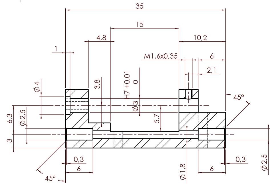
COUPE A-A ECHELLE 3 : 1
