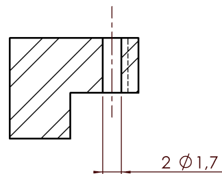
COUPE B-B ECHELLE 3 : 1
